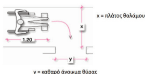
Σχήμα 5: Στροφή χρήστη αναπηρικού αμαξιδίου κατά 90°
